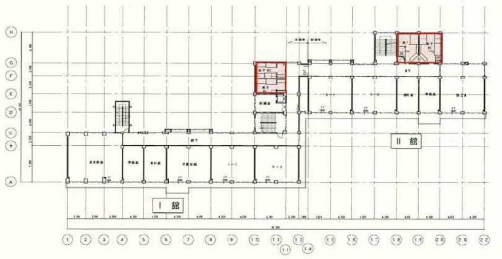
門沢橋小学校 4階平面図
