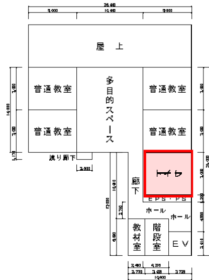
4階平面図
