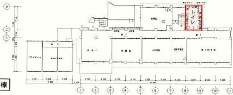
海西中学校 1階平面図
