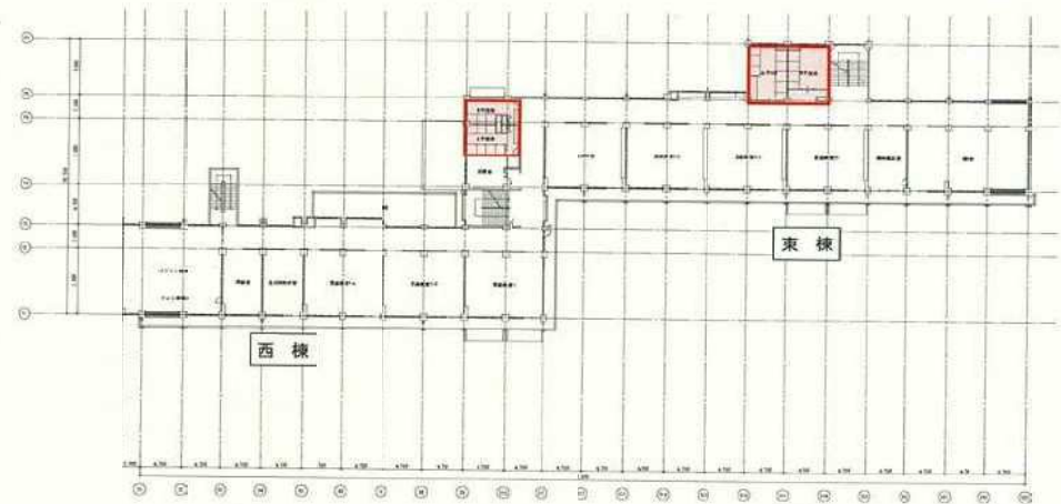
中新田小学校 2階平面図
