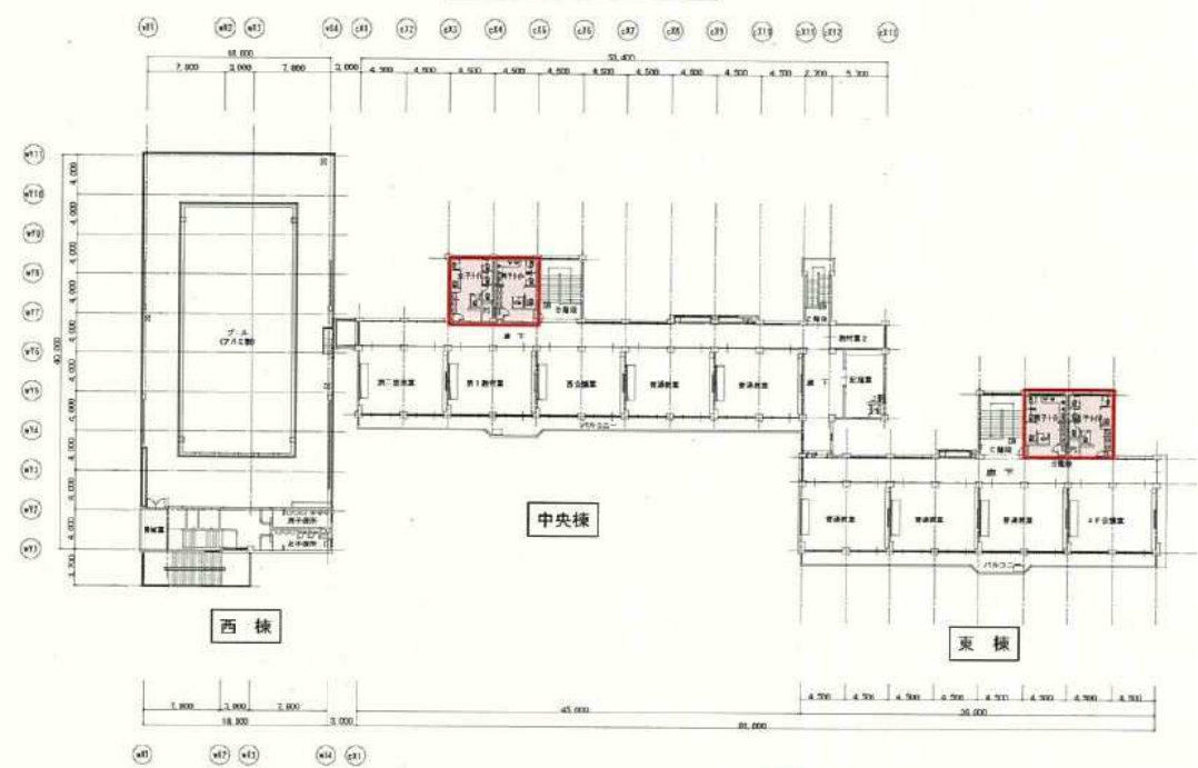
大谷中学校 4階平面図
