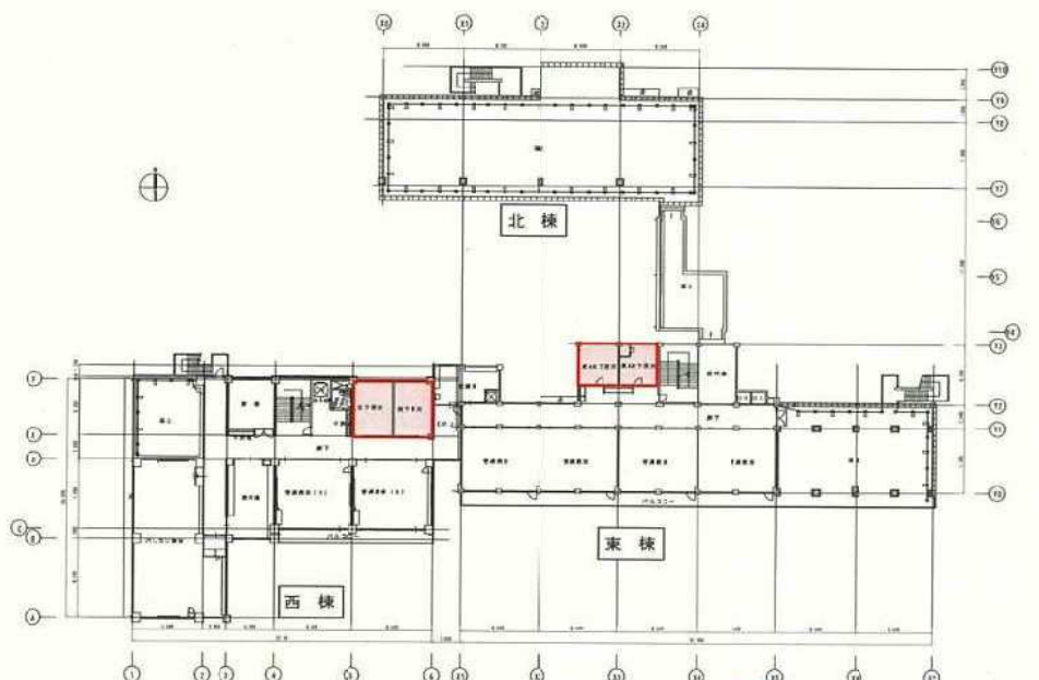
海老名小学校 4階平面図
