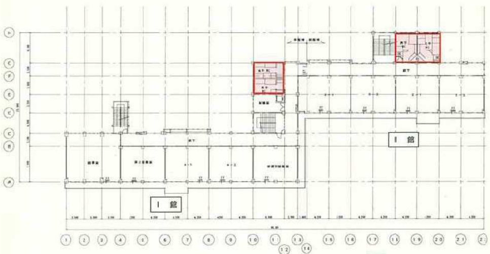
門沢橋小学校 3階平面図
