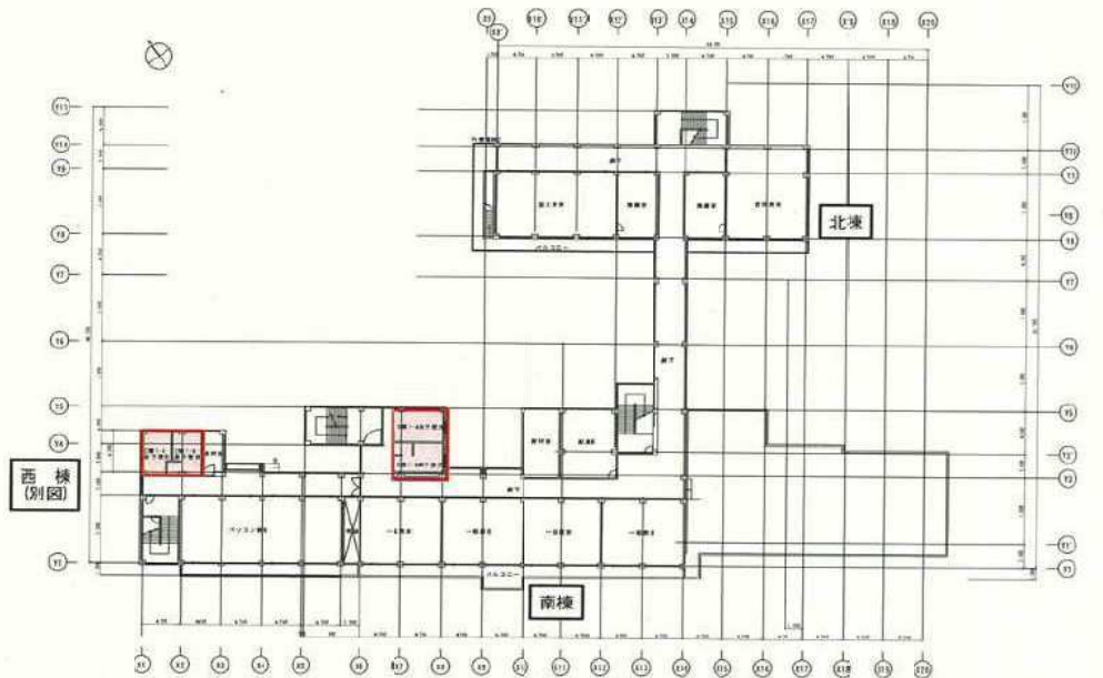
今泉小学校 4階平面図
