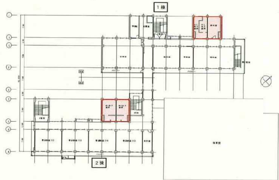
杉本小学校 4階平面図
