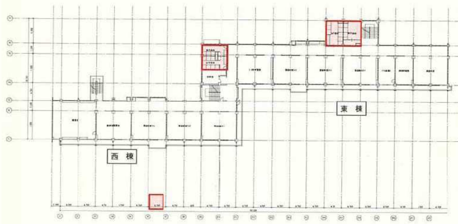
中新田小学校 3階平面図
