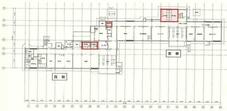
中新田小学校 1階平面図
