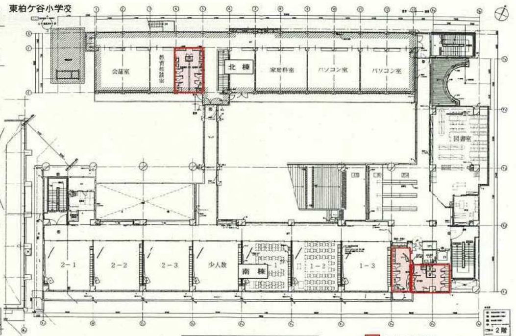
東柏ケ谷小学校 2階平面図
