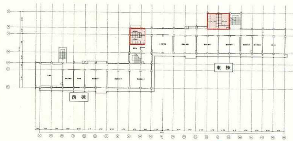
中新田小学校 4階平面図
