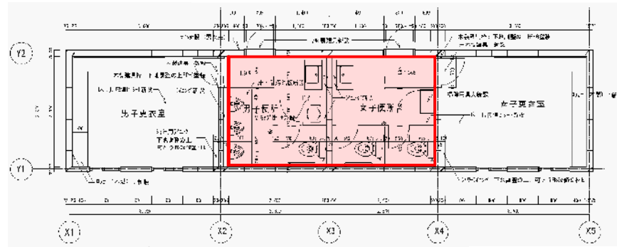
屋内運動場付属棟 平面図
