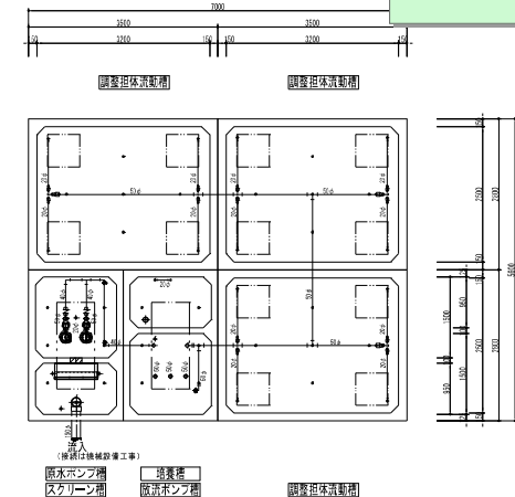
スラブ下平面図 1/50 (消泡ポンプ配管)
