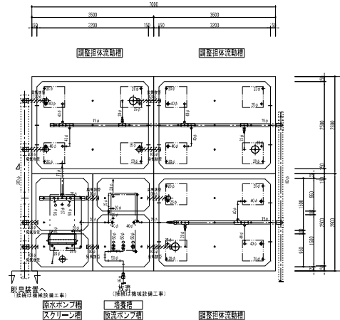
スラブ平面図 1/50 (エア配管)
