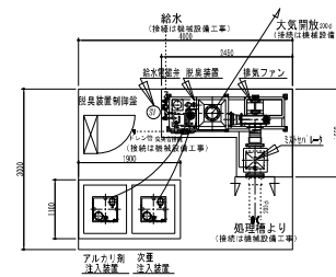
脱臭装置設備スペース図 (屋上設置)
