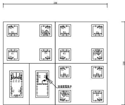
エア配管図 1/50
