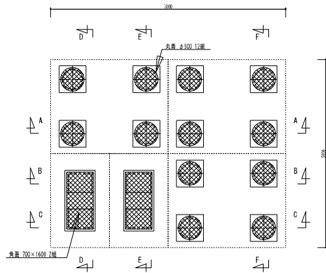
頂板開口部図 1/50
