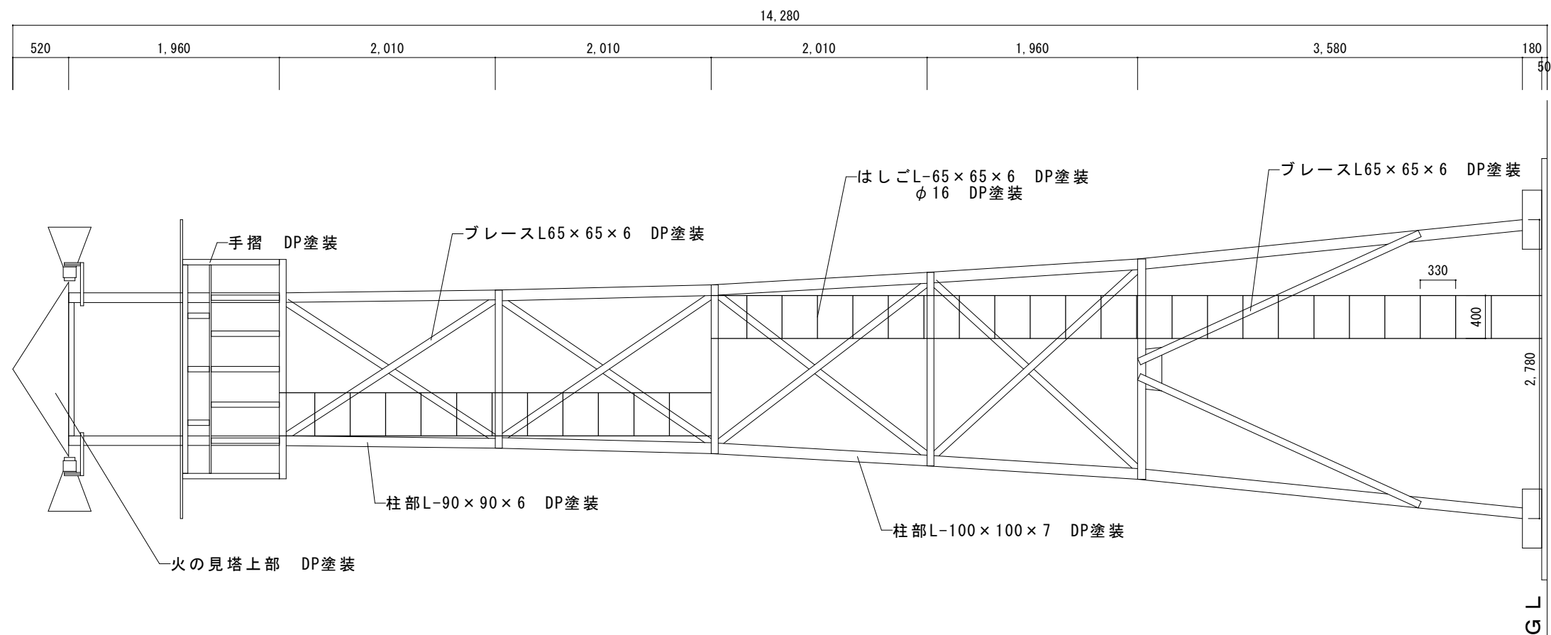
立面図
