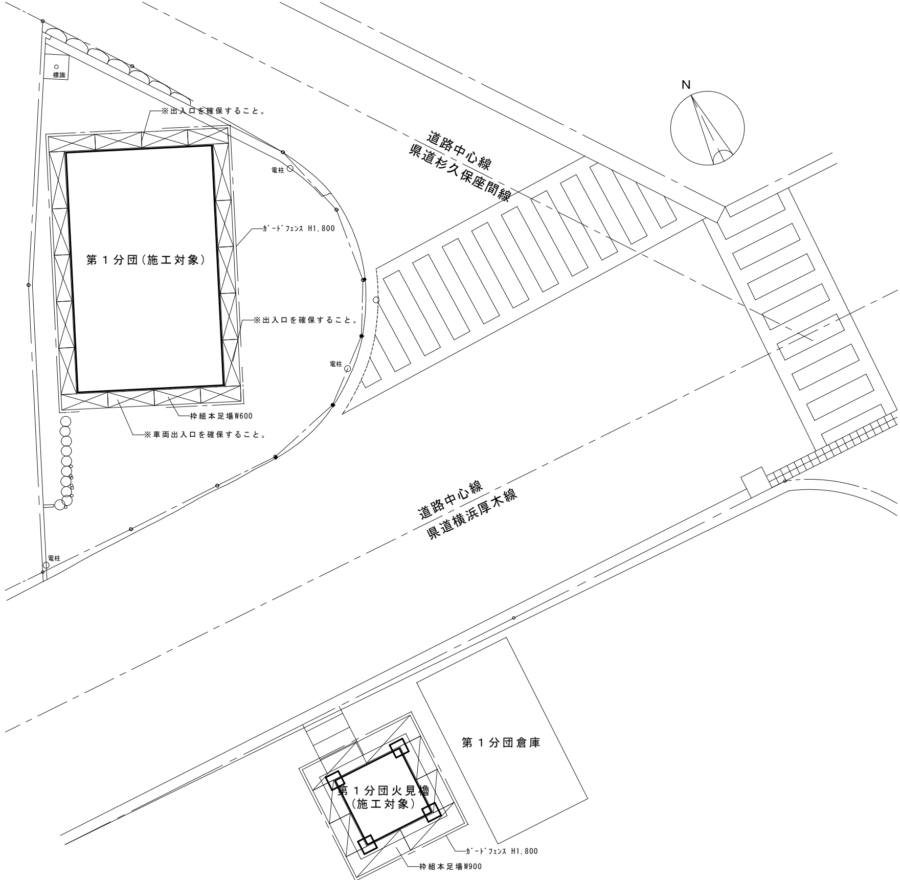
配置図兼仮設計画図(参考)
