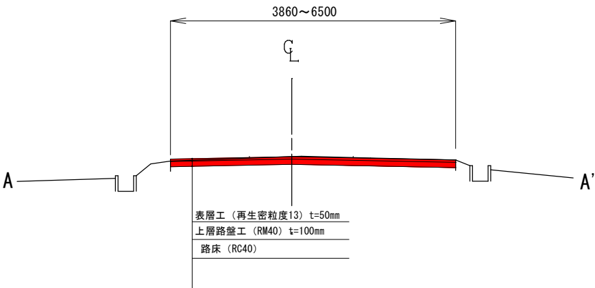
標準横断面
