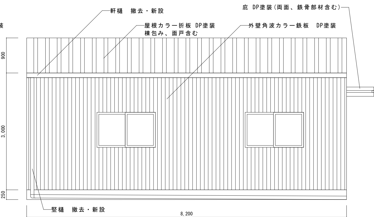
北側立面図
