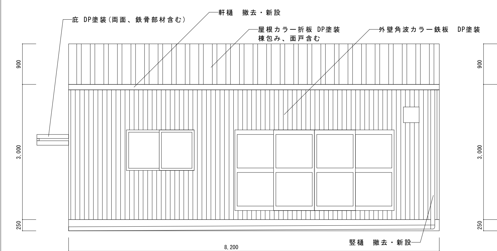
南側立面図
