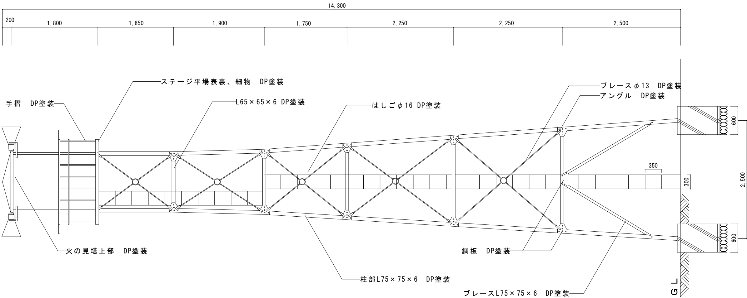
立面図
