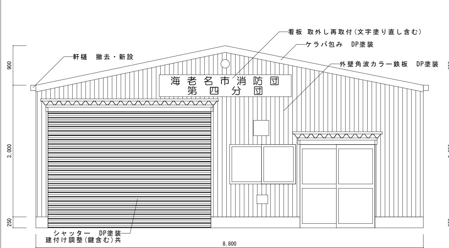
西側立面図
