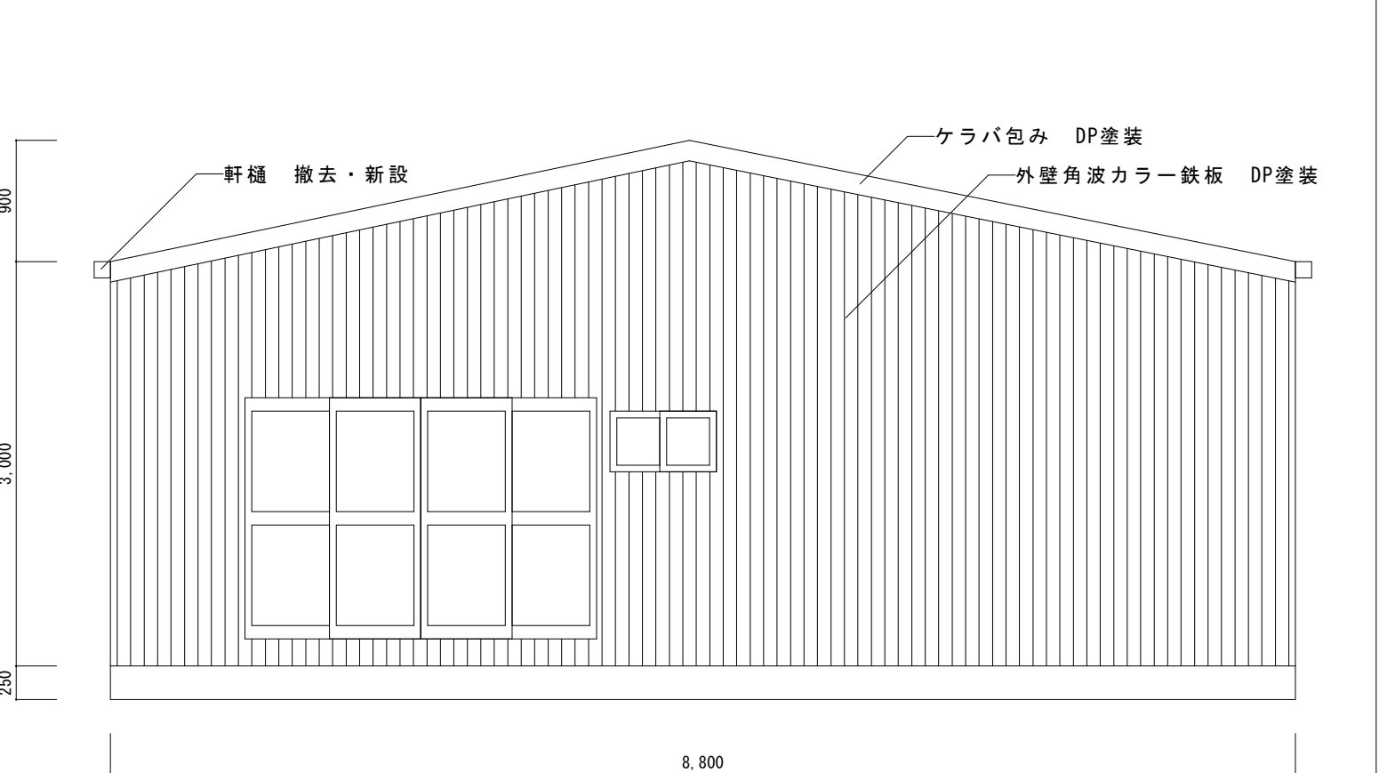
東側立面図
