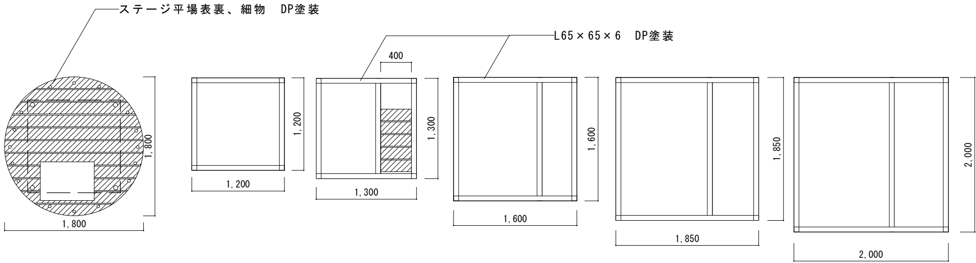
平面図
