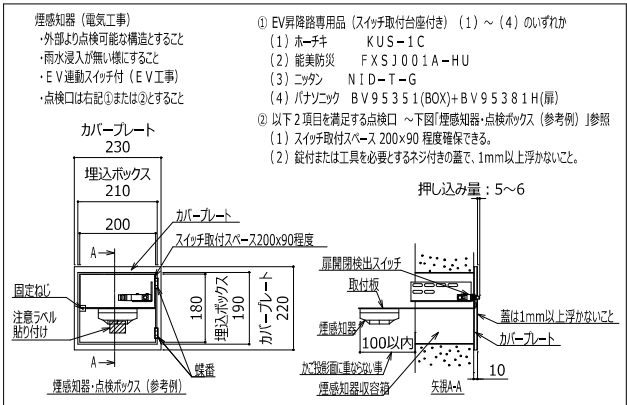
煙感知器施工例
