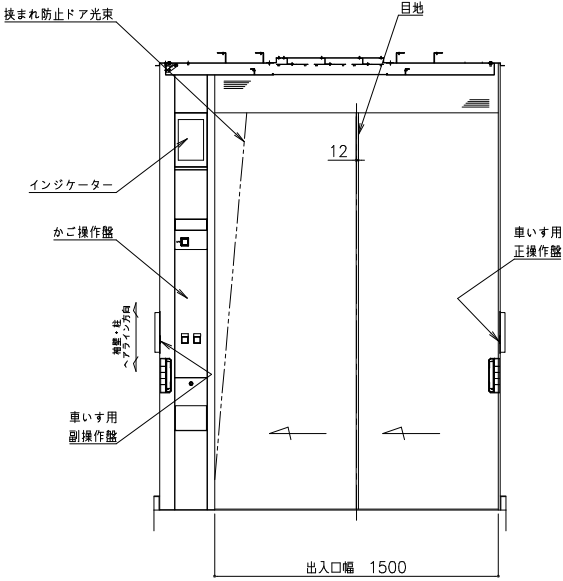
かご室正面図（矢視A-A）
