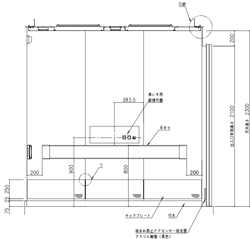
かご室側面図（矢視B-B）
