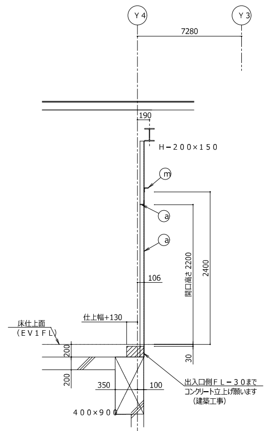
Y-Y断面
