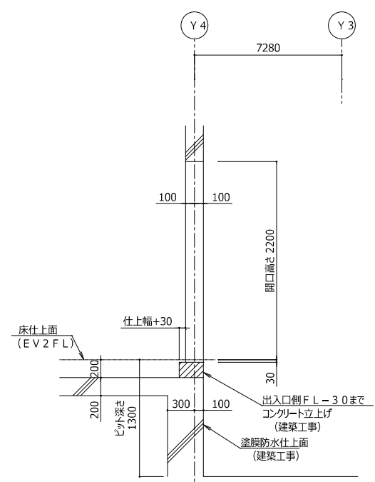
X-X断面
