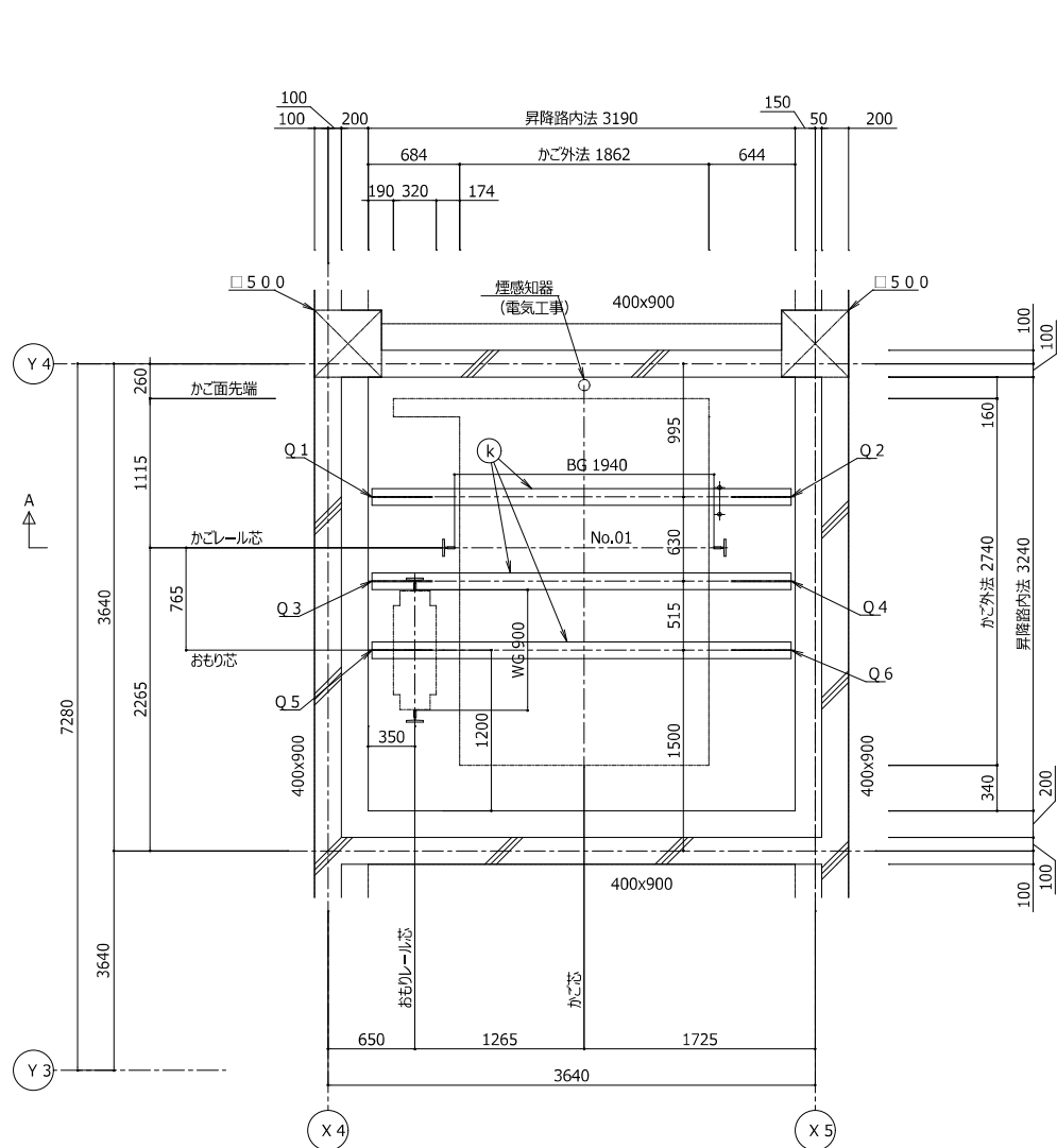
昇降路平面図 (1/30) (頂部)
