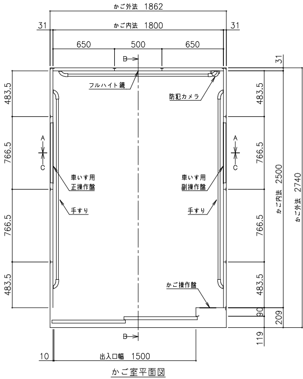
かご室平面図
