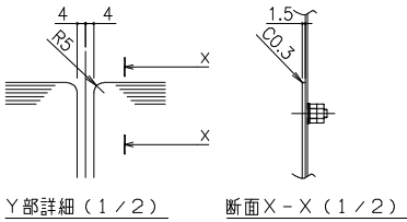
Y部詳細（1／2）
