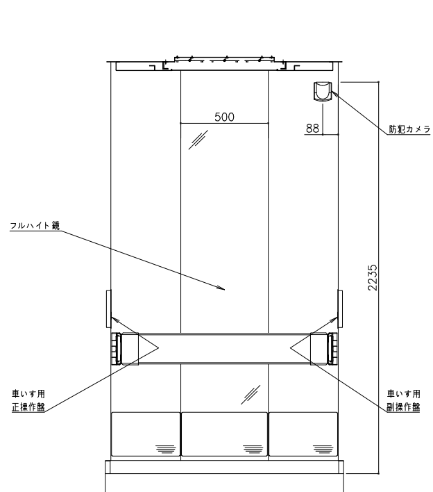
かご室背面図（矢視C-C）
