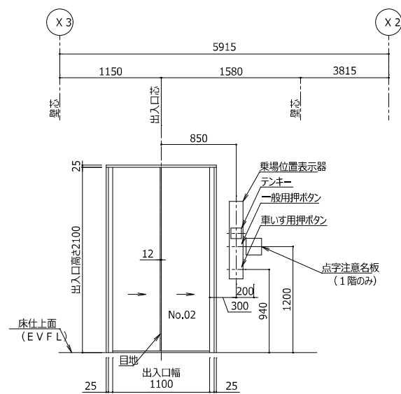
乗場正面図 (1/30) (No. 02号機) (1、2階)
