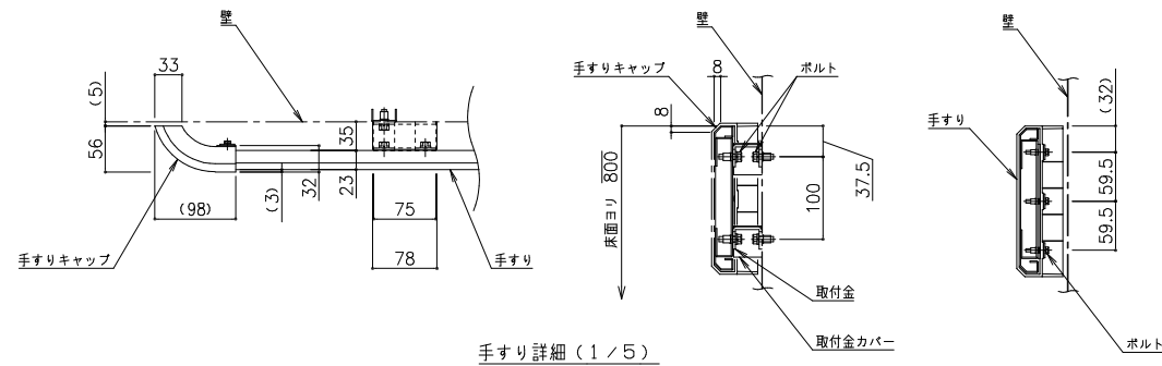
手すり詳細（1/5）
