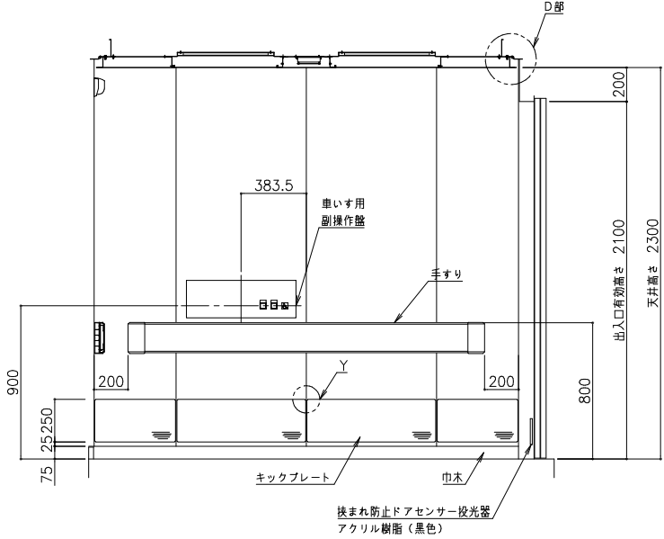
かご室側面図（矢視B-B）
