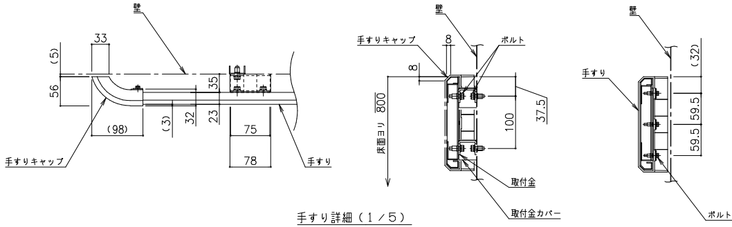
手すり詳細（1／5）
