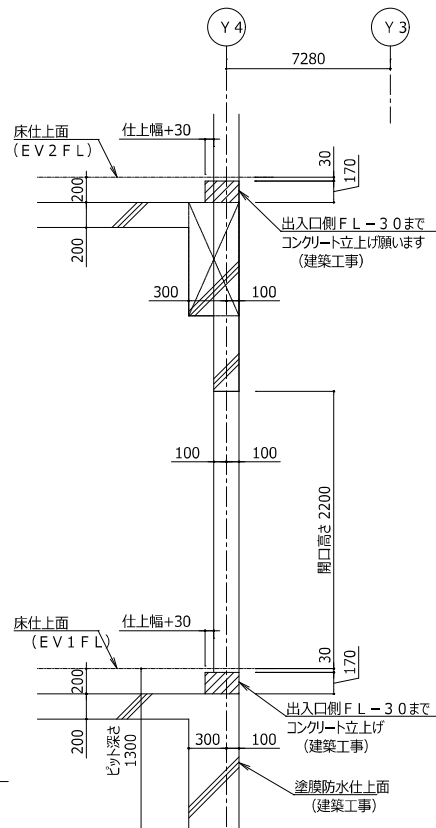
X-X断面
