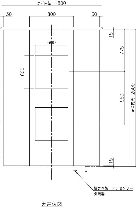
天井伏図
