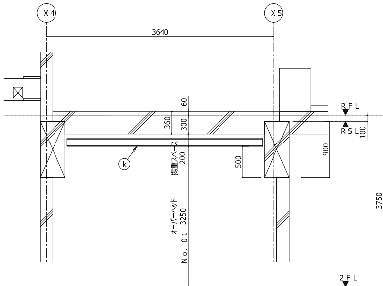
昇降路頂部断面図 (1/30) 断面 A-A
