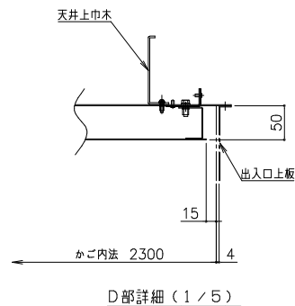
D部詳細（1/5）
