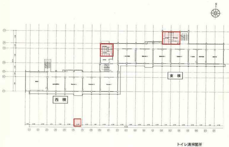
中新田小学校 3階平面図
