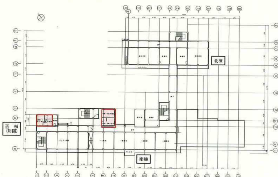
今泉小学校 4階平面図
