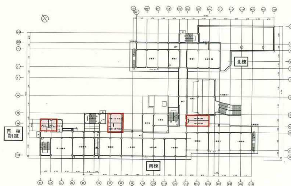
今泉小学校 2階平面図
