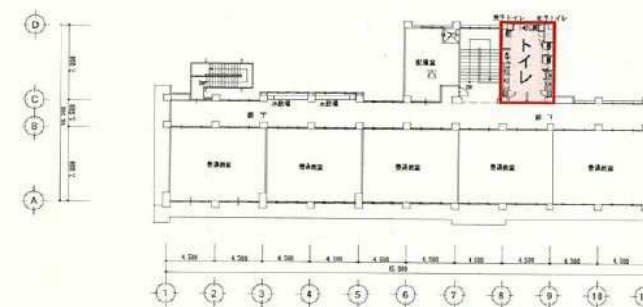
海西中学校 4 階平面図
