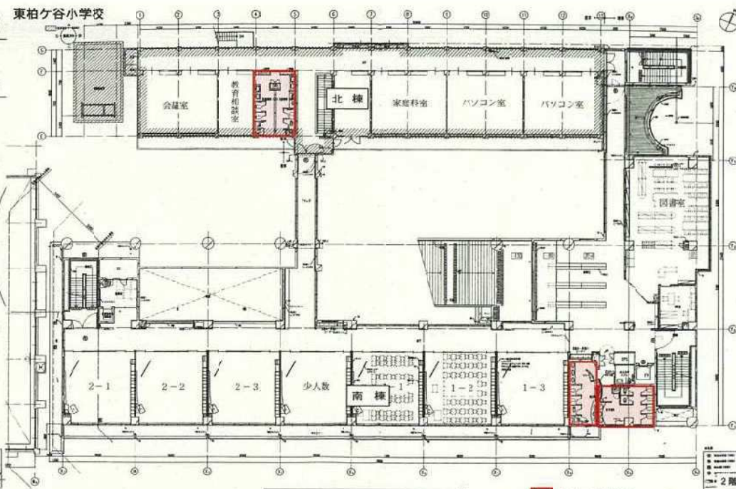
東柏ケ谷小学校 2階平面図
