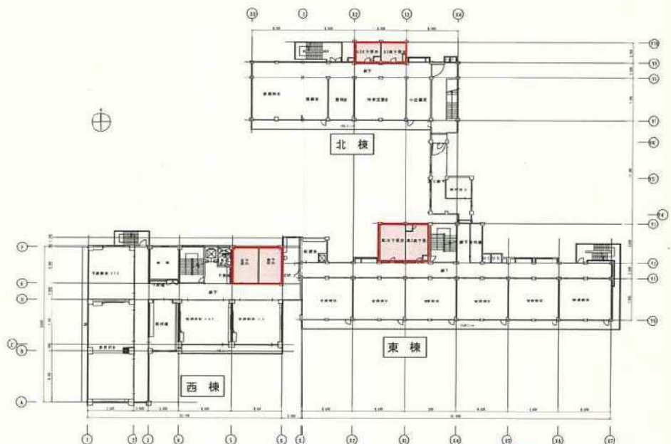
海老名小学校 3階平面図
