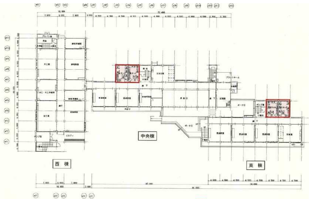
大谷中学校 1階平面図
