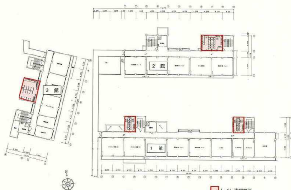
上星小学校 2階平面図
