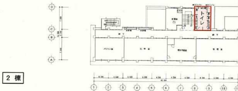
海西中学校 2 階平面図
