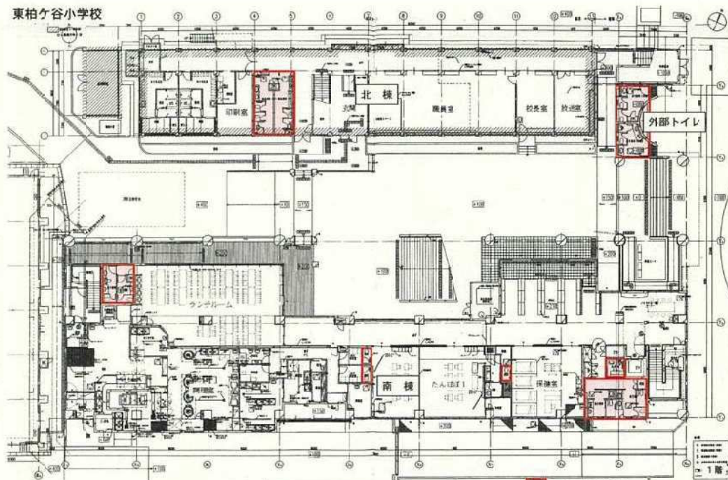
東柏ケ谷小学校 1階平面図
