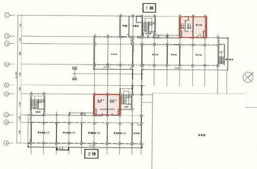
杉本小学校 4階平面図
