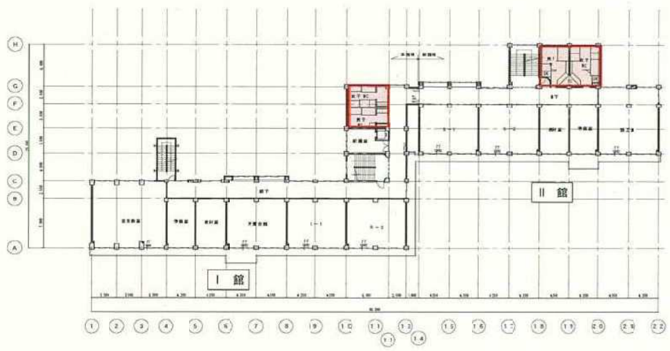
門沢橋小学校 4階平面図
