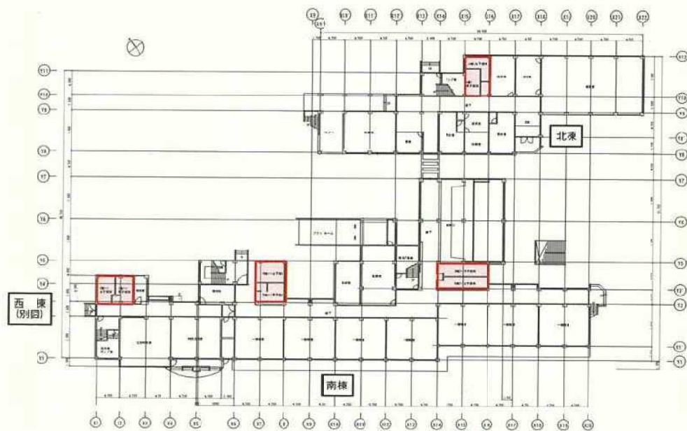
今泉小学校 1階平面図
