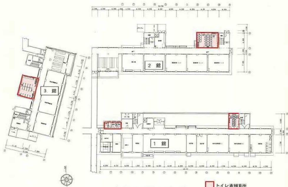
上星小学校 1階平面図
