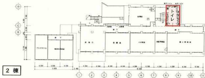
海西中学校 1 階平面図
