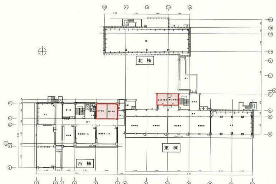
海老名小学校 4階平面図
