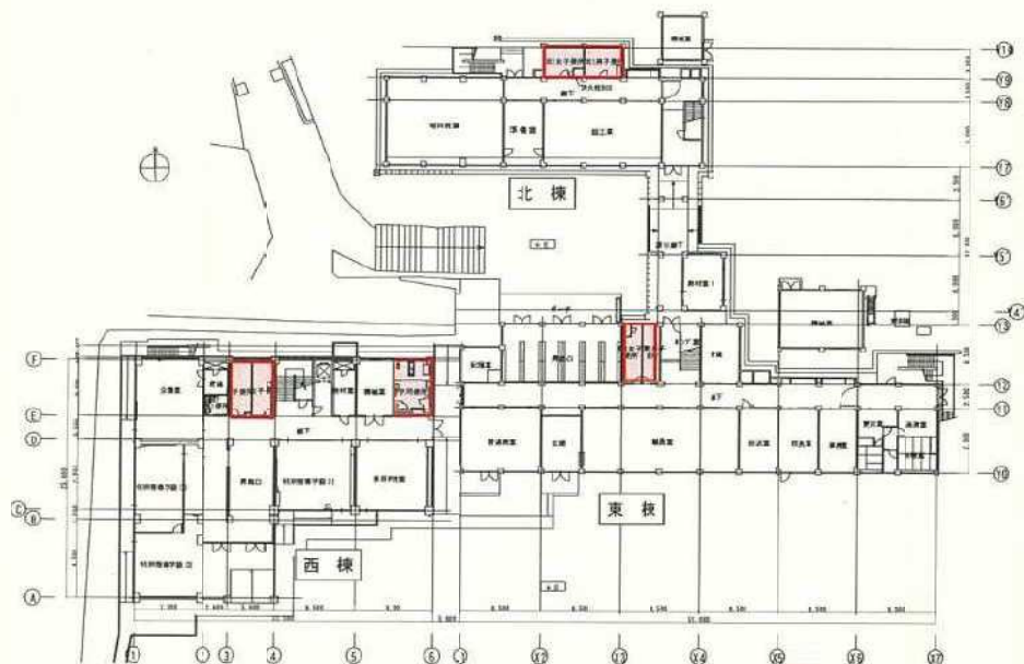
海老名小学校 1階平面図
