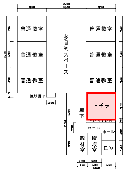
3 階平面図
