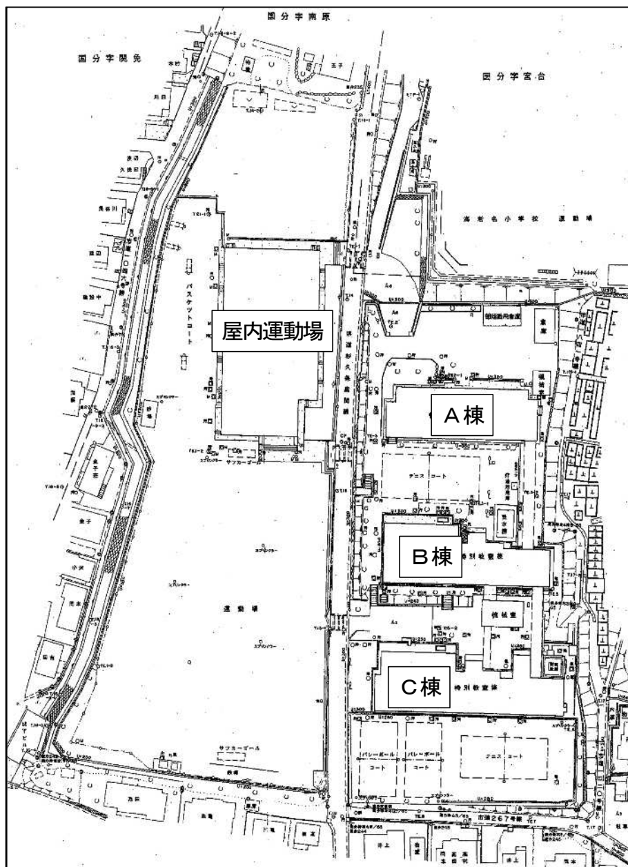
海老名中学校 配置図
