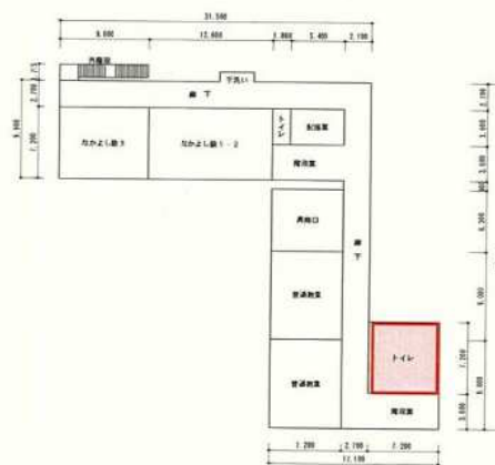
東館 1階平面図
