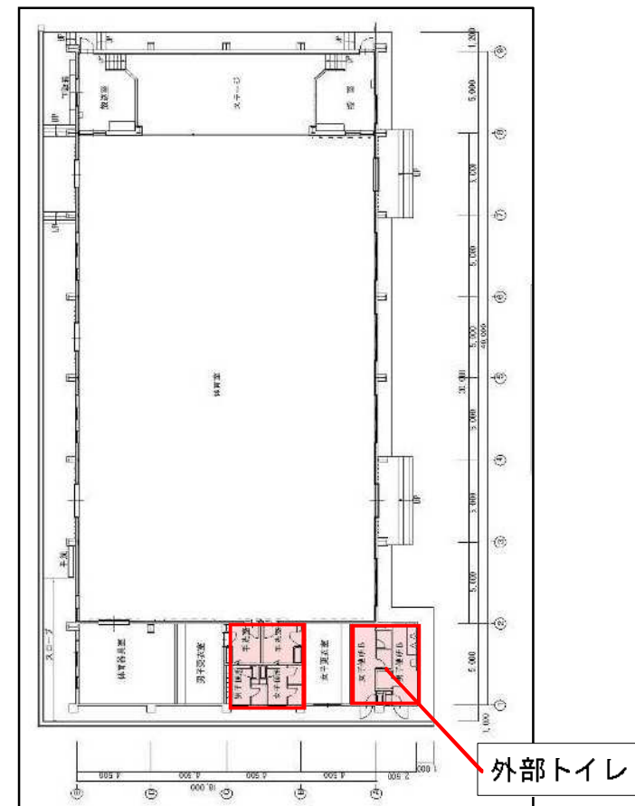
屋内運動場 平面図
