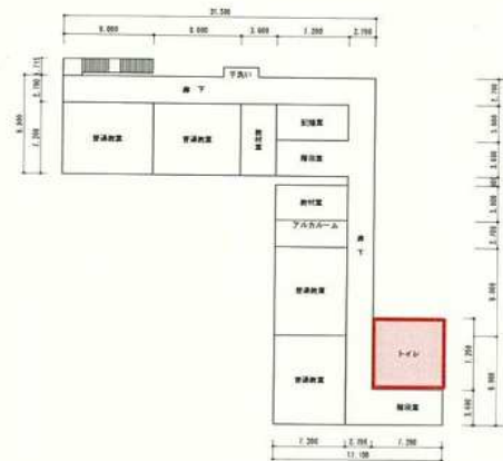
東館 2階平面図
