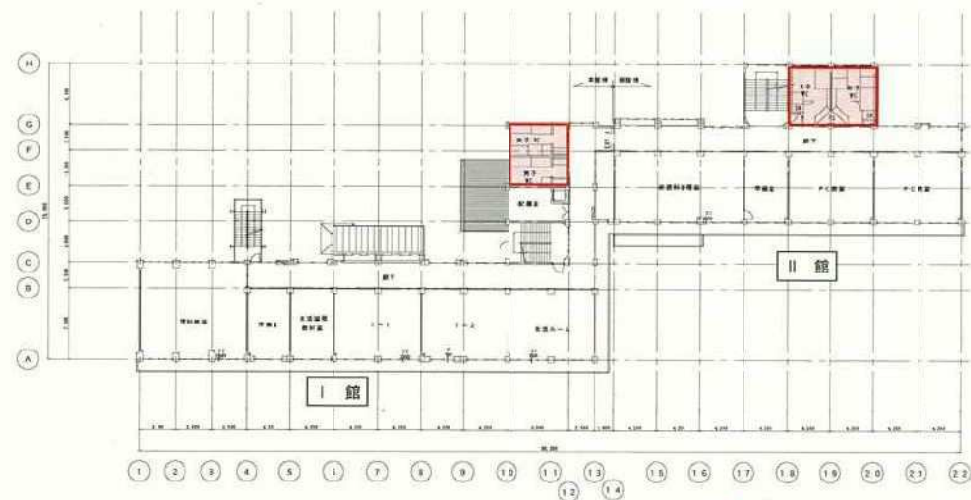
門沢橋小学校 2階平面図
