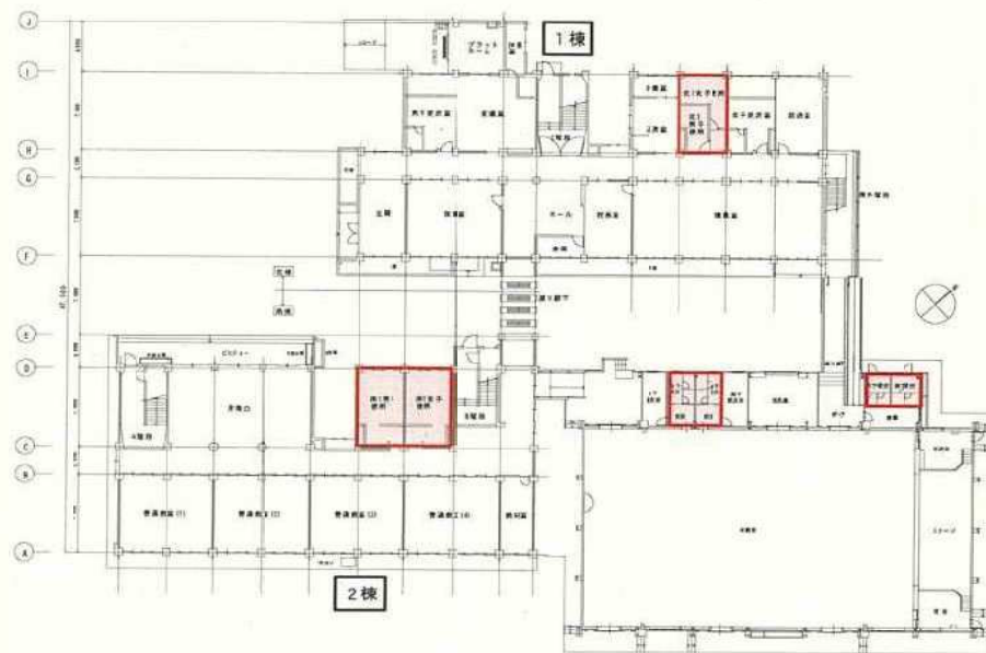
杉本小学校 1階平面図
