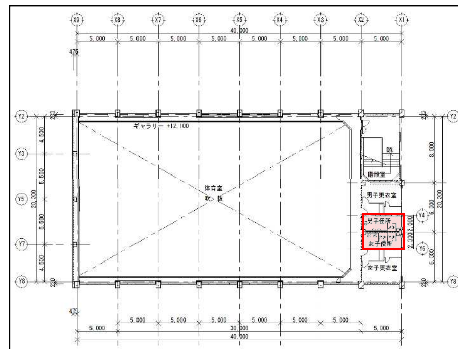
屋内運動場 4階 平面図
