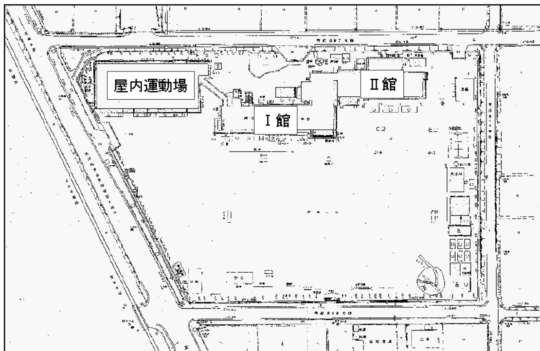
門沢橋小学校 配置図
