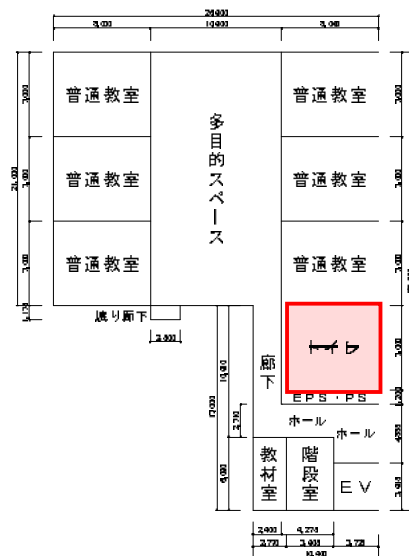
2 階平面図
