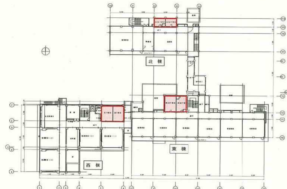
海老名小学校 2階平面図
