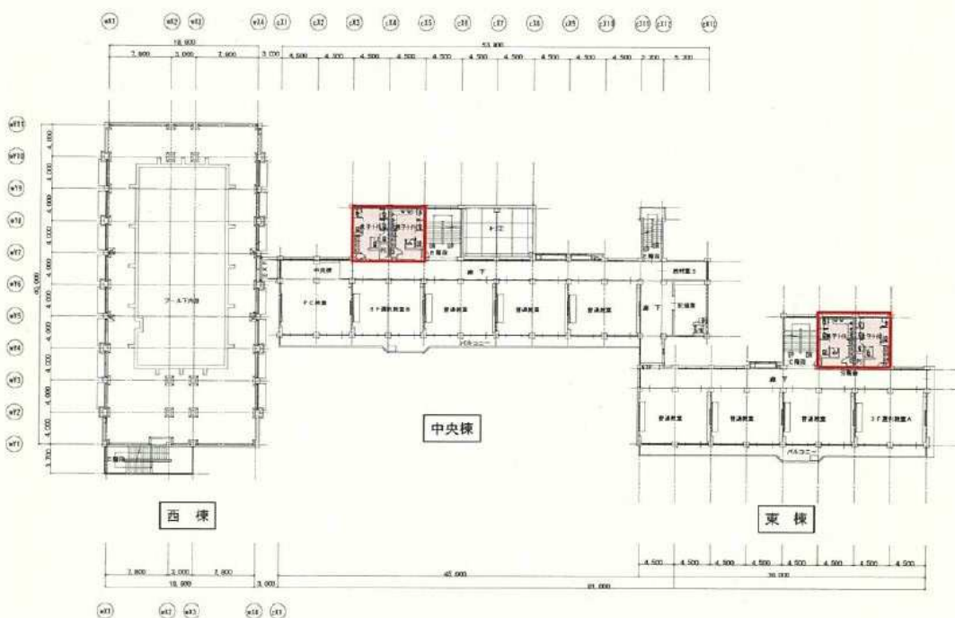
大谷中学校 3階平面図
