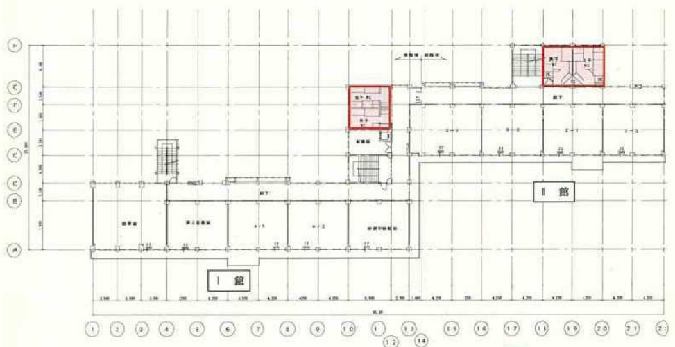
門沢橋小学校 3階平面図
