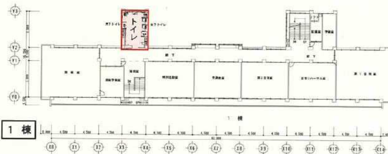
海西中学校 2 階平面図
