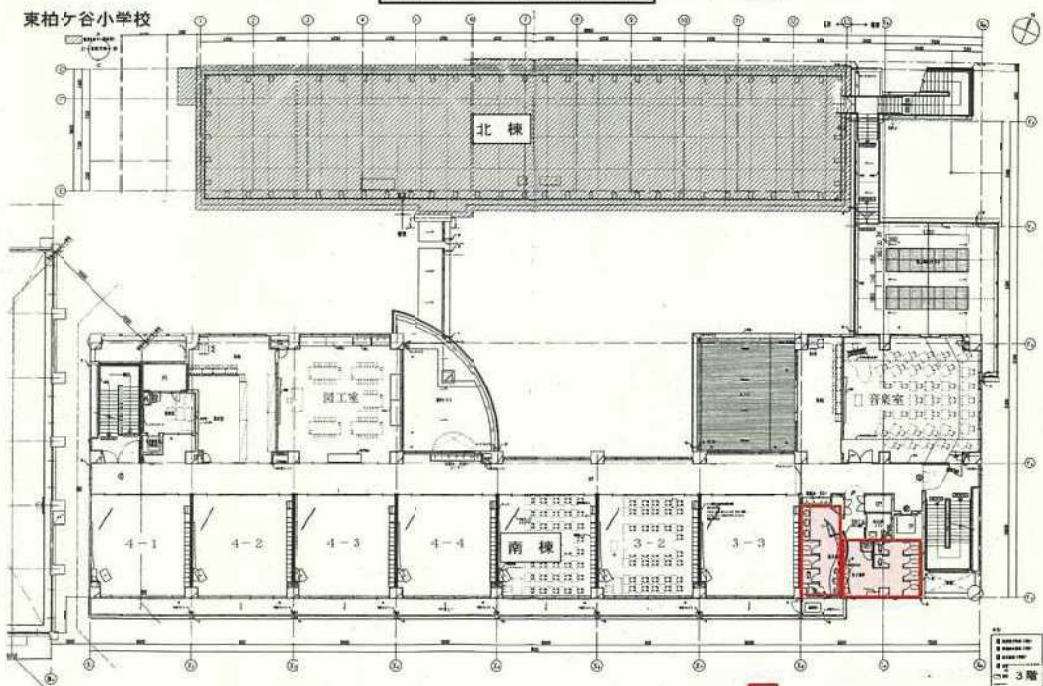
東柏ケ谷小学校 3階平面図
