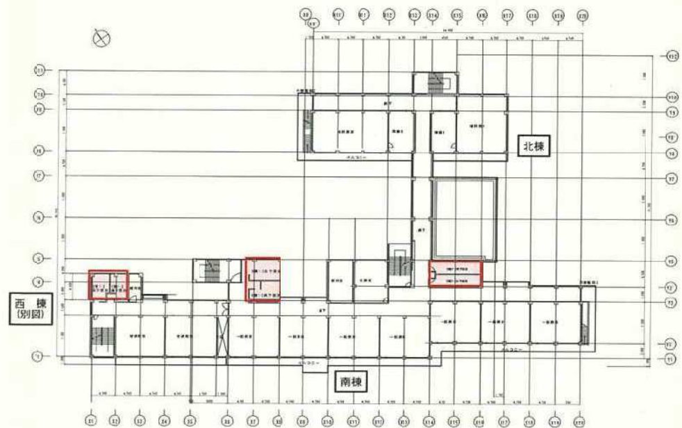
今泉小学校 3階平面図
