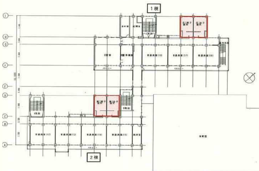
杉本小学校 3階平面図
