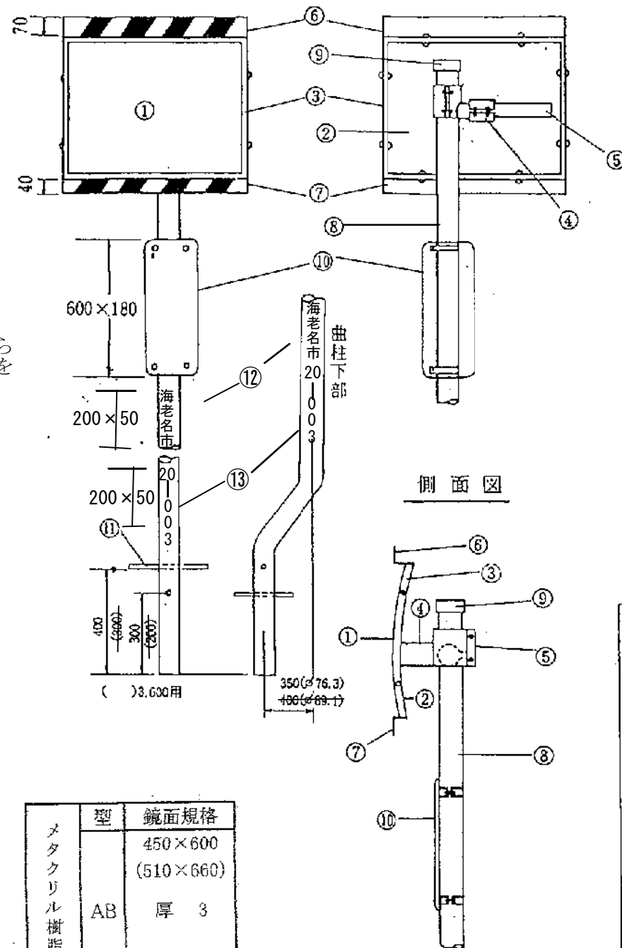
正面図
