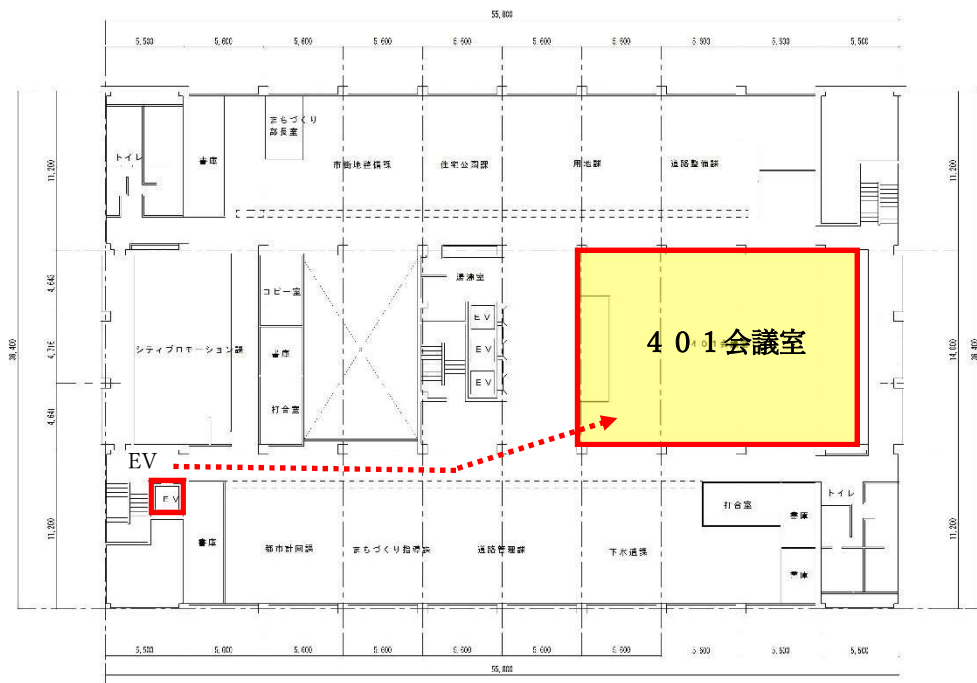
海老名市庁舎4階平面図 1/200
