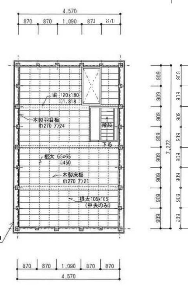
〔2階平面図〕
