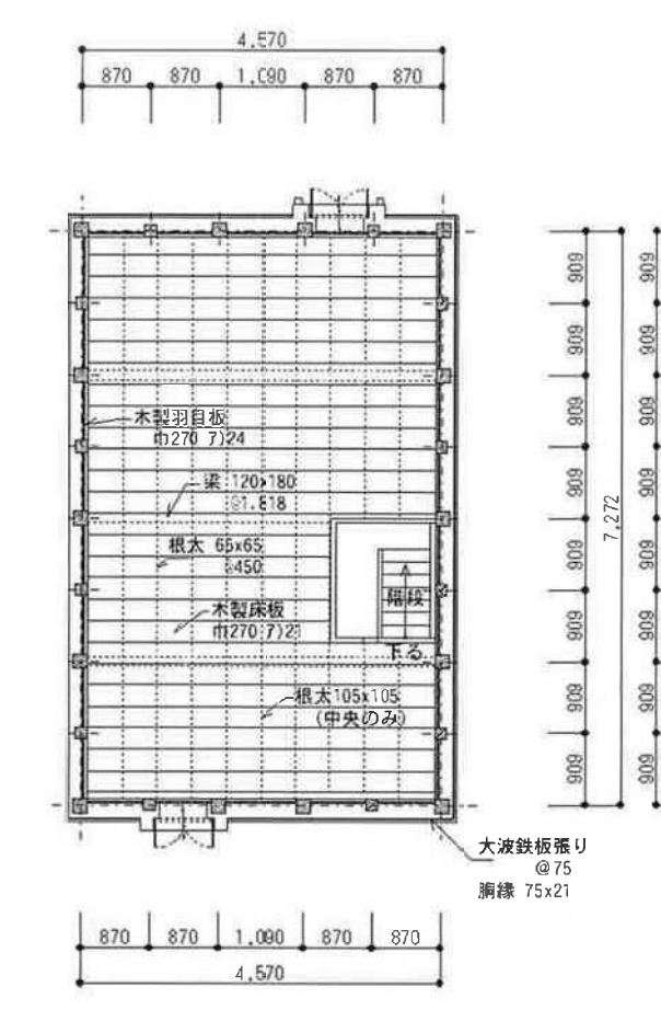
〔3階平面図〕
