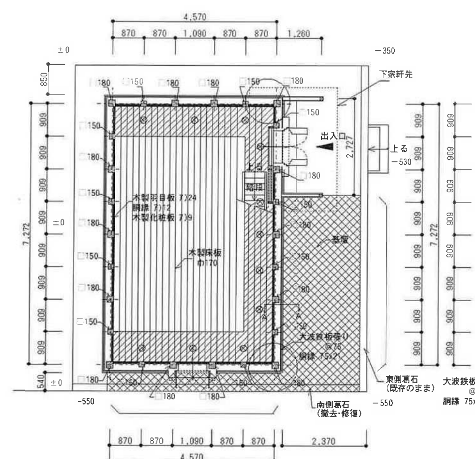
〔1階平面図〕
