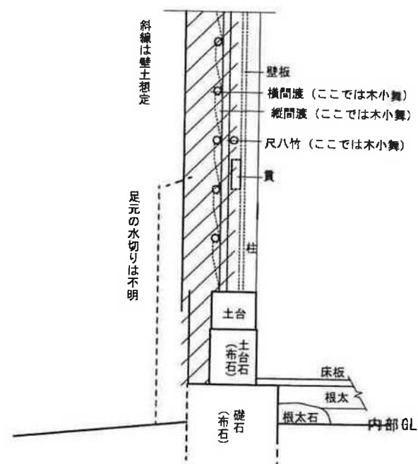
建立時推定断面
