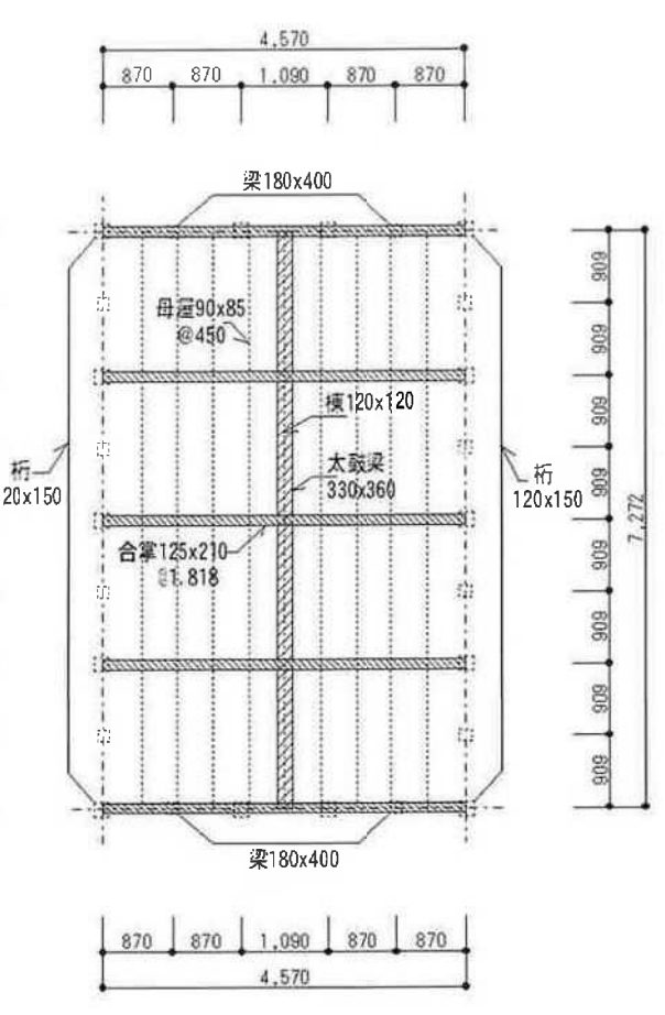
〔小屋伏図〕
