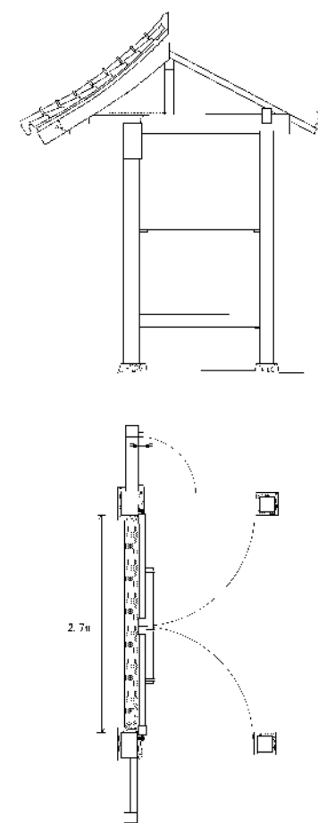
薬医門断面図・平面図
