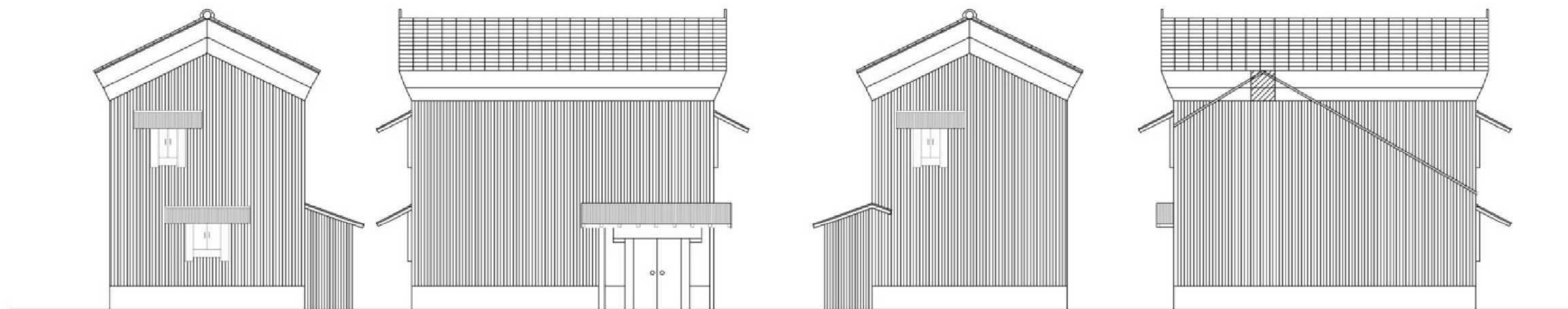
南側立面図
