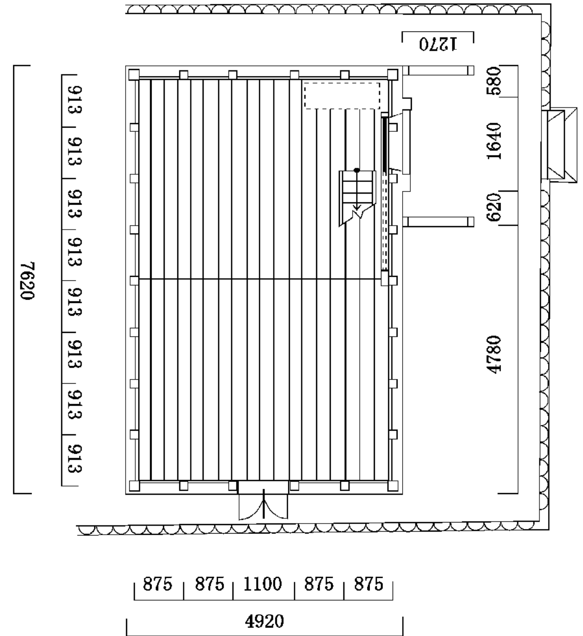
1 階平面図
