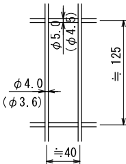
ワイヤメッシュ図 ( ) 内は芯径を示す。
