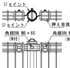
A部取付図 S=1:10
