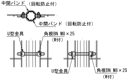
標準的な取付図 パネルと柱のすきまがせまい場合の取付図
