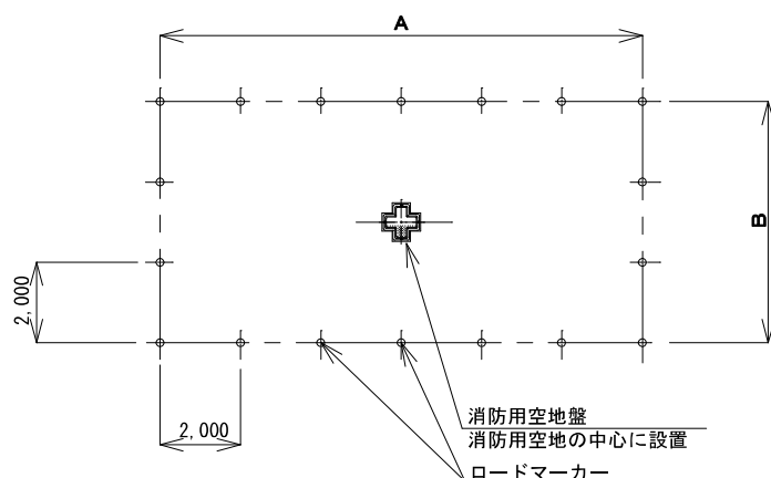
【 ロードマーカース設置寸法 】
