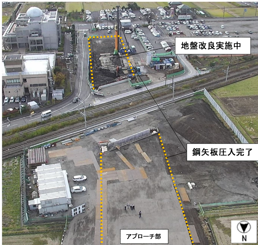
【JR相模線北側工事ヤードより(ドローン撮影)】
