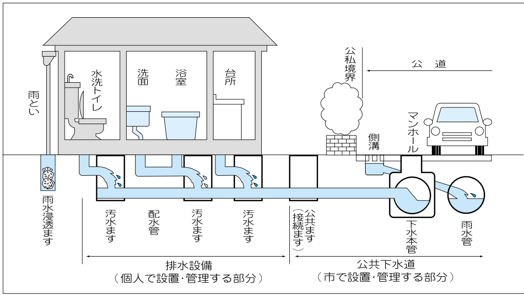
水洗化工事の一例(一般家庭の場合)
