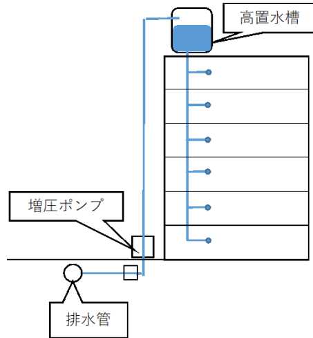
増圧直結高置水槽方式
