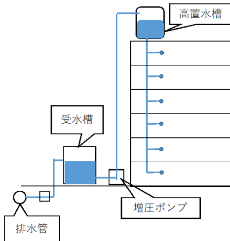
受水槽高置水槽方式
