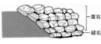
▲葺石状基壇
