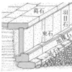
▲壇上積基壇
