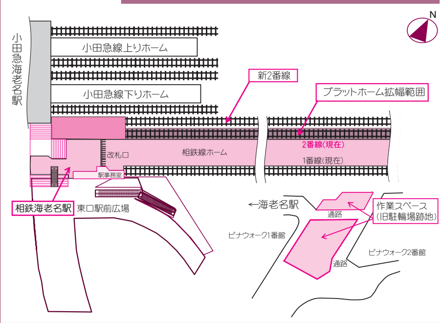
相鉄線海老名駅ホーム拡幅工事概略図
